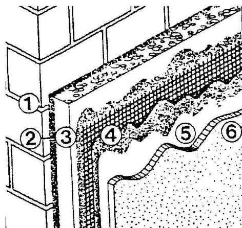
Obr. 1 Příklad jednoplášťového zateplovacího systému
