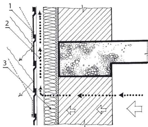
Obr. 2 Příklad dvouplášťového zateplovacího systému
