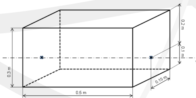
Obrázek 1 – Výklenek pro umístění vodoměru s uvedenými minimálními rozměry
